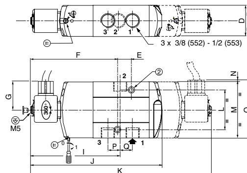
TYPE 06: WBLP Metal cap/PBT EN/IEC 60079-7, EN/IEC 60079-18 and EN/IEC 61241-1
