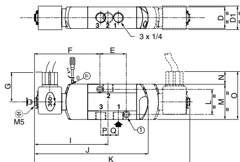
TYPE 05: WBLP Metal cap/PBT EN/IEC 60079-7, EN/IEC 60079-18 and EN/IEC 61241-1
